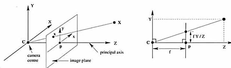
Figura 7 - Modelo geométrico da câmera Pinhole. Fonte: Hartley e Zisserman (2004)
