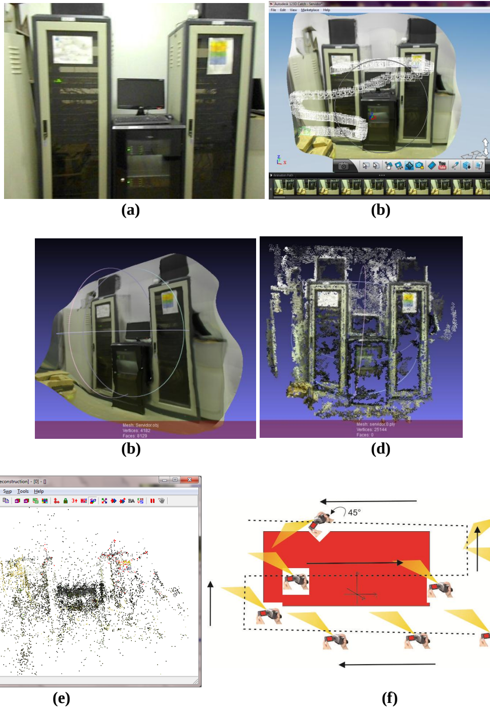
Figura 33 – Reconstrução Servidor.
