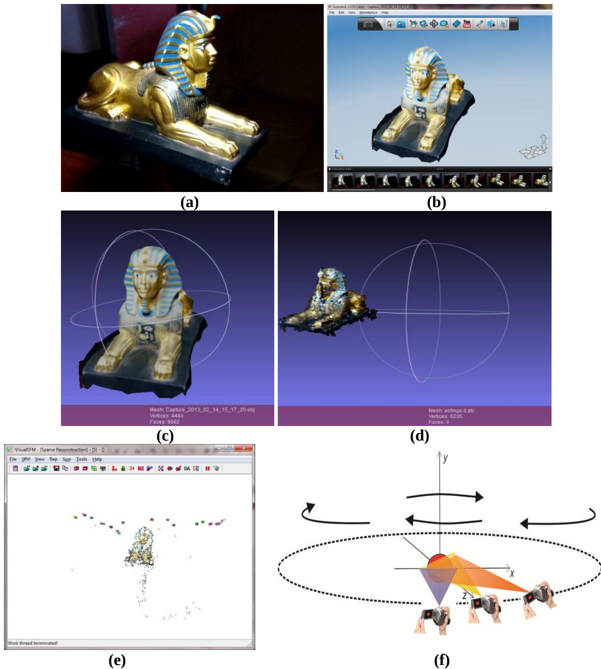
Figura 30 – Reconstrução Esfinge.
