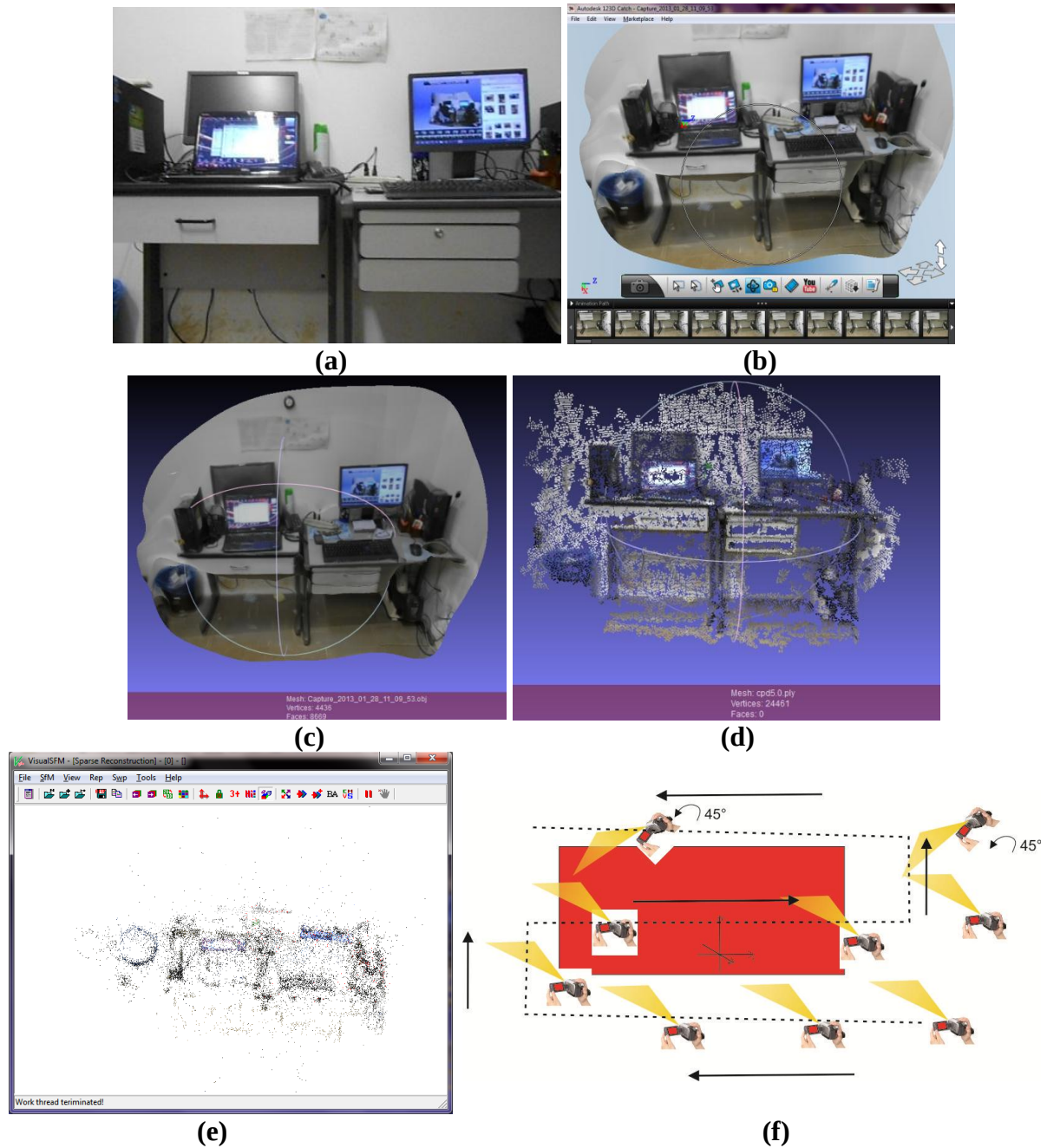
Figura 32 – Reconstrução CPD.
