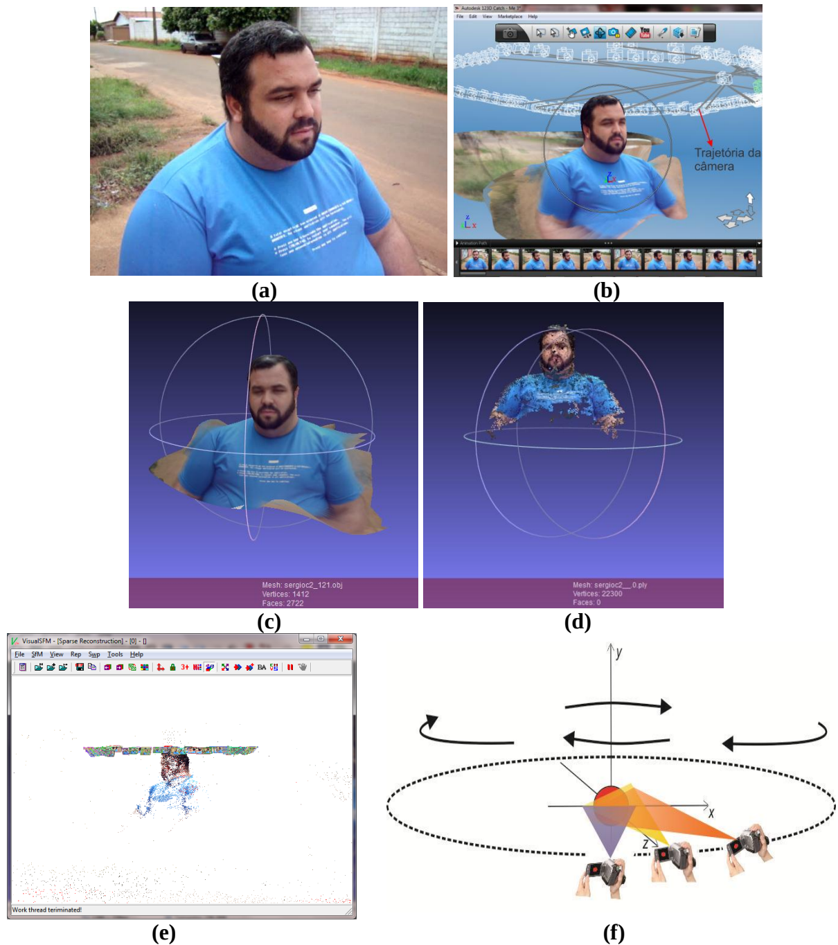
Figura 31 – Reconstrução Sergio.
