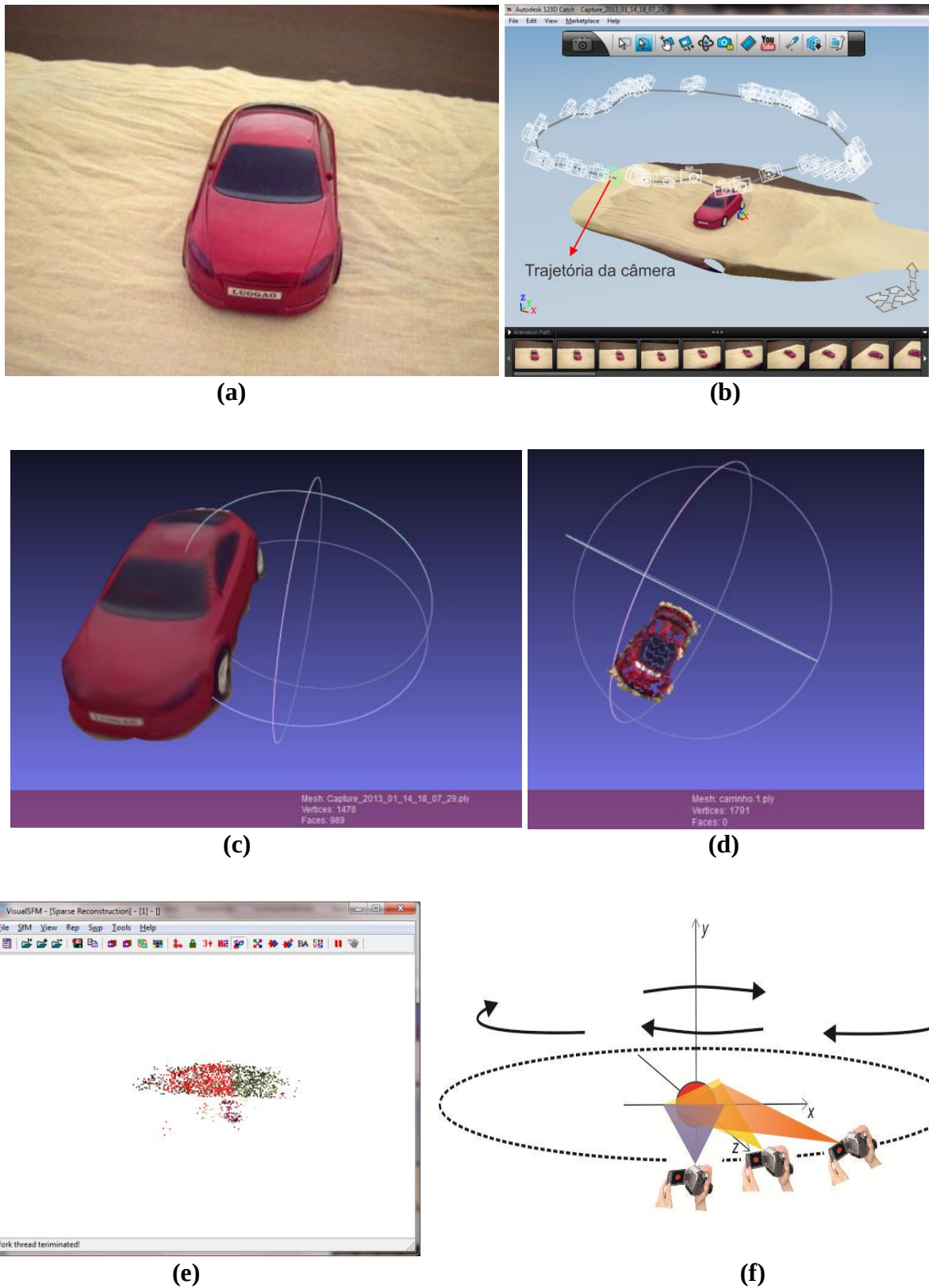
Figura 29 – Reconstrução Carrinho.
